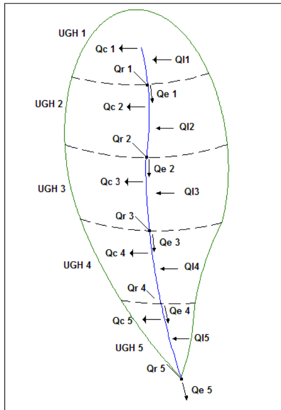
Figura 2 - Vazões características nas UGHs de uma bacia hidrográfica hipotética.
