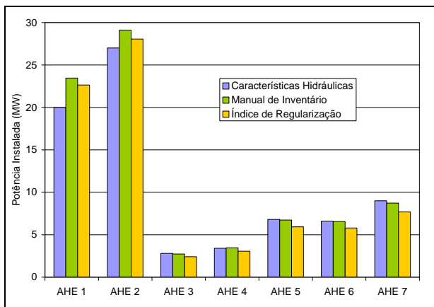
Figura 8 – Potências de dimensionamento determinadas pelos diferentes métodos.
