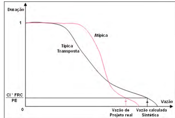
Figura 7 - Relação duração entre hidrologias de comportamento distinto.
