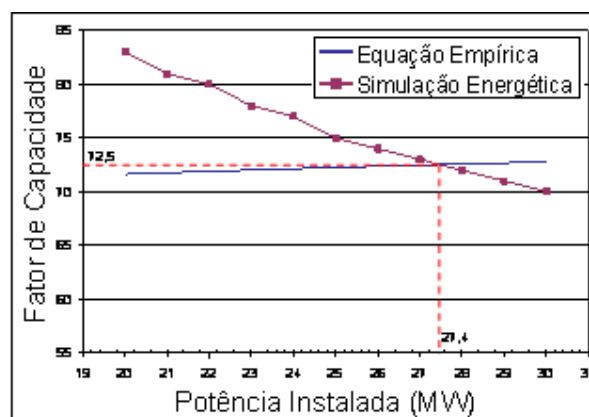
Figura 5 – Identificação do fator de capacidade de referência pelo método das características hidráulicas.
