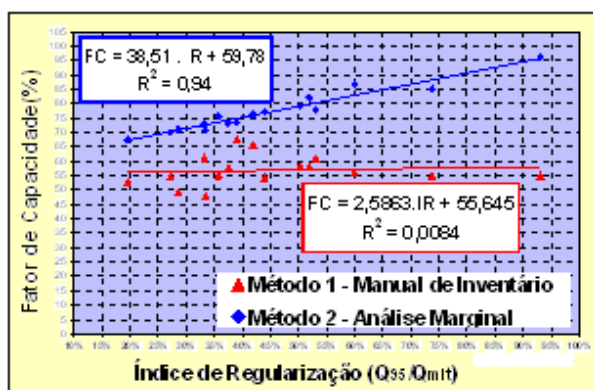
Figura 1 – Fator de capacidade em função do índice de regularização.
